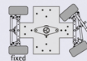
後輪ステアリング
