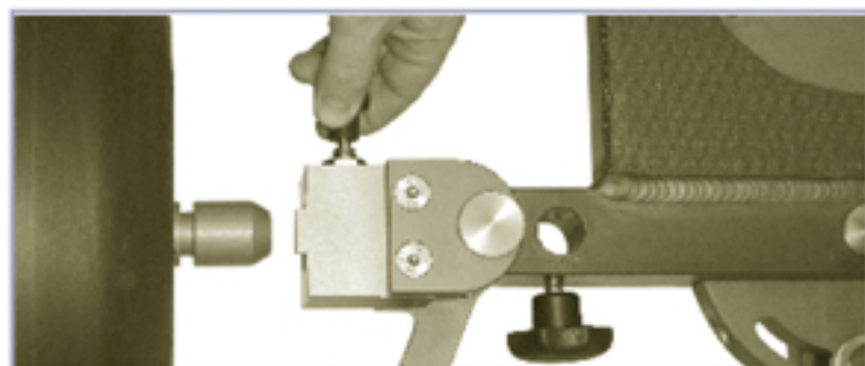
迅速なホイール取り外し
