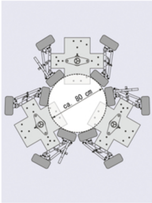
極めて小さい回転範囲 (80cm)
