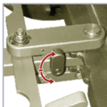
ステアリングモード切り替え
